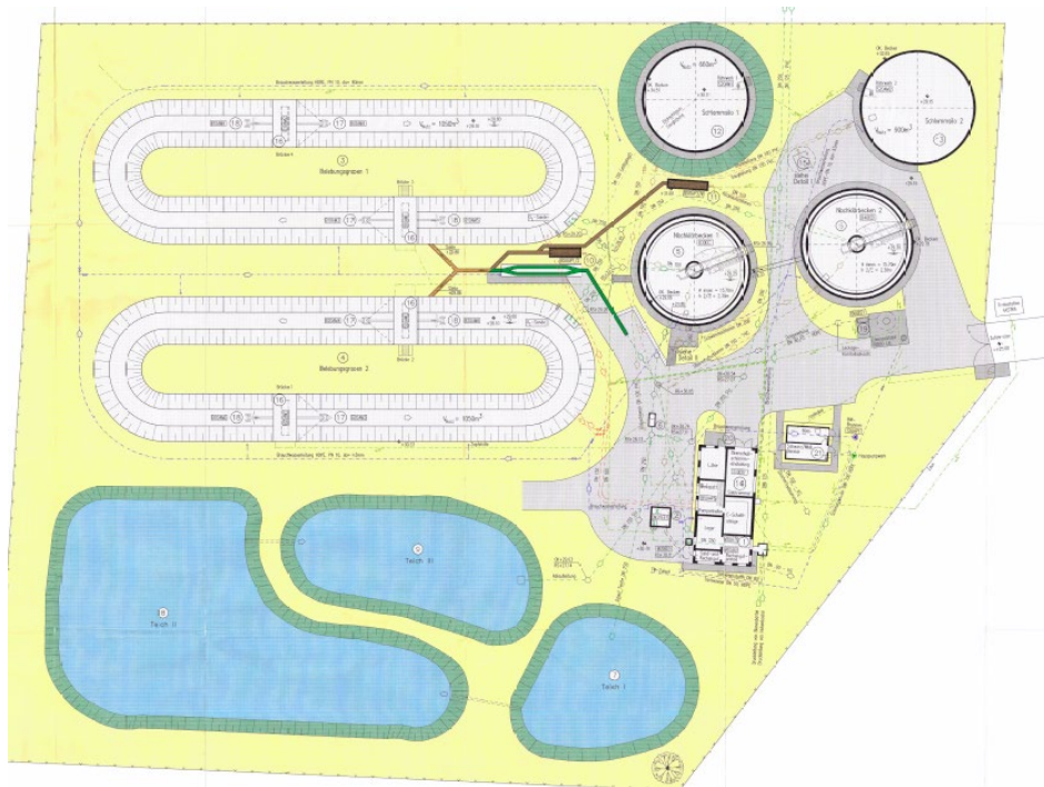
Abbildung 3-2: Lageplan KA Bienenbüttel Bestand
