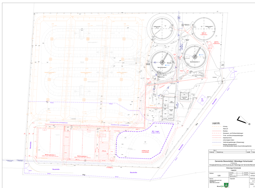
Abbildung 4-2: Lageplan der Kläranlage Bienenbüttel mit geplanten Maßnahmen 2
